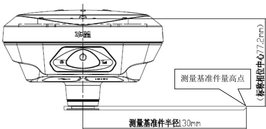
图 2-10 量高示意图
